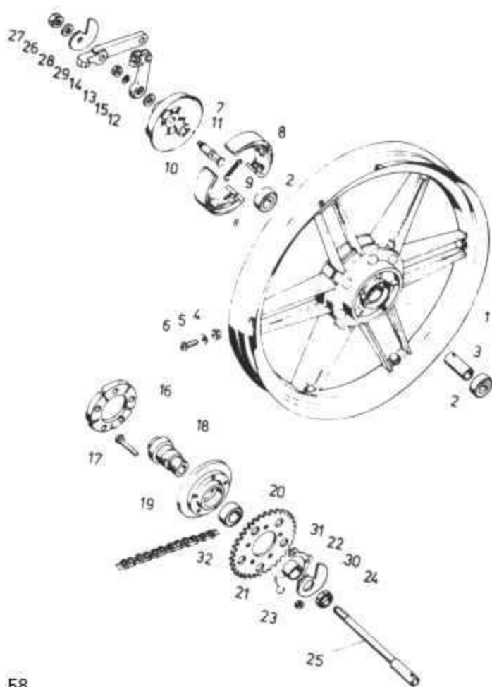
afb. 58 - achtersterwiel
