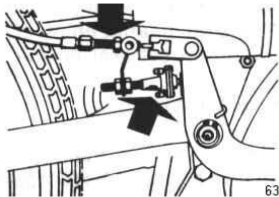
afb. 63 - afstellen trommelrem
