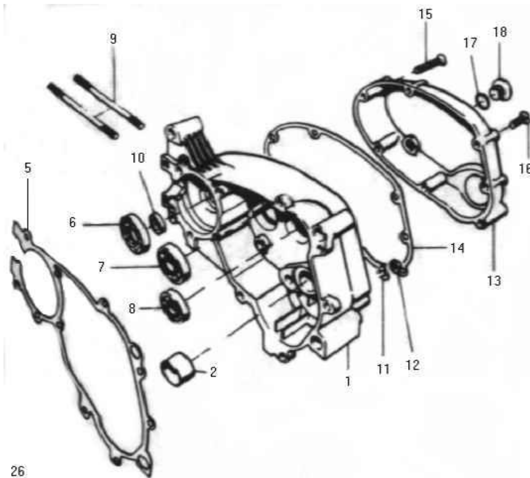
afb. 26 - carterhelft rechts (alle typen 4 versn.)
