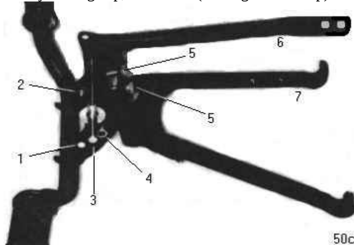
afb. 50c - hulpframe
