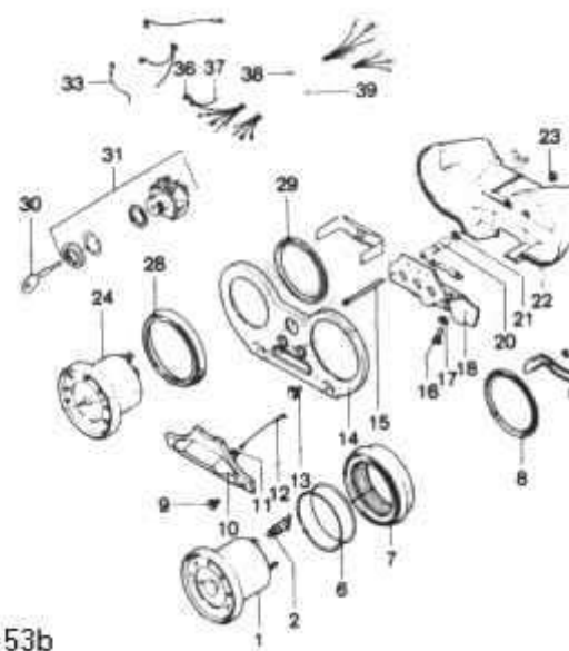
afb. 53b - cockpit
