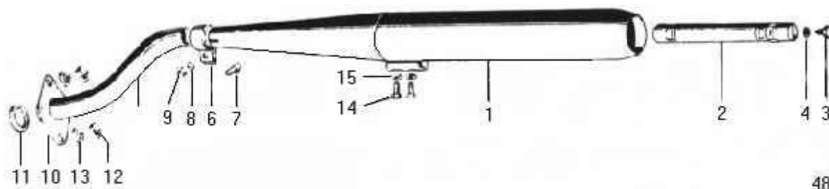
afb. 48 - uitlaatsysteem
