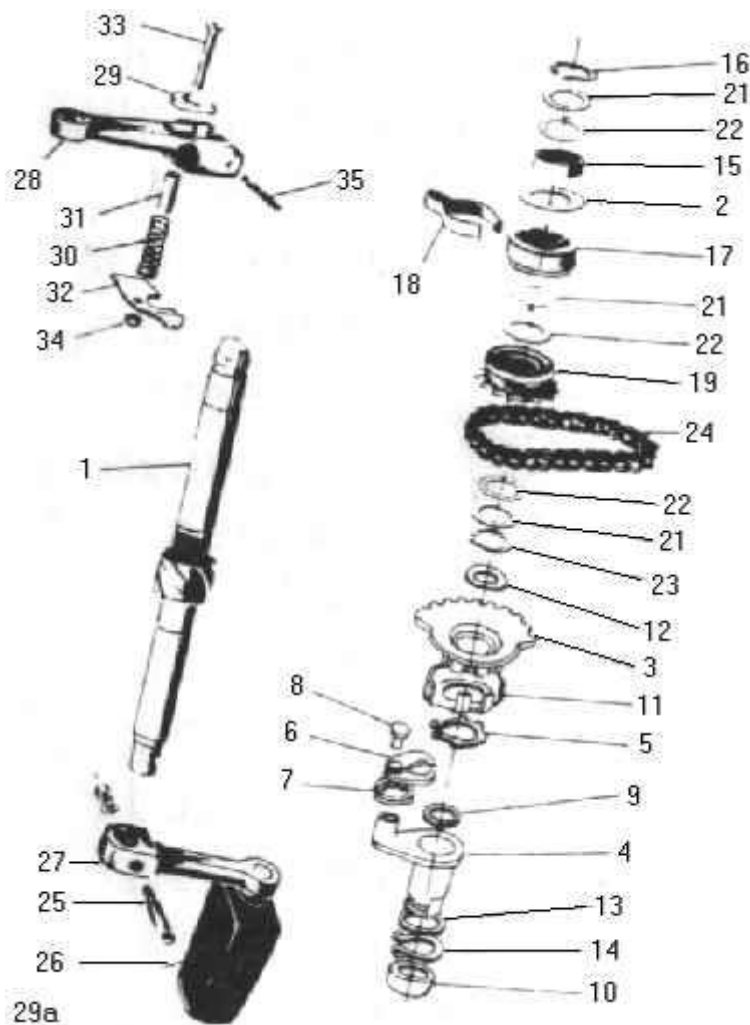
afb. 29a - trapmechanisme (4 versn.bak indirecte schakeling)
