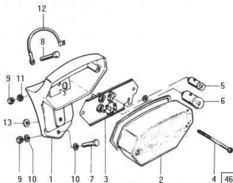
afb. 46 - achterlicht
