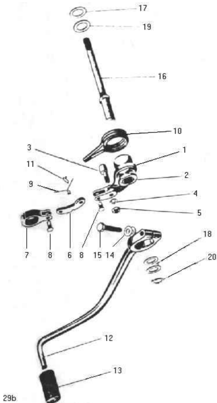
afb. 29b - schakelset (4 versn.bak indirecte schakeling)
