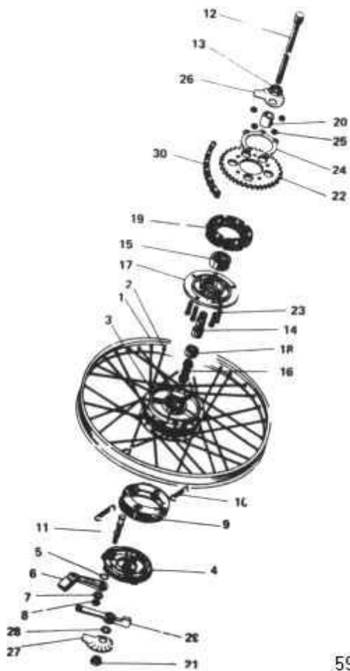
afb. 59 - achterspaakwiel
