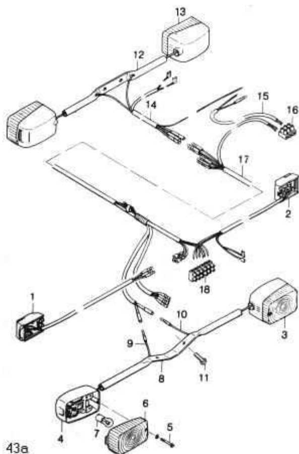
afb. 43a - clignoteurs en schakelaar
