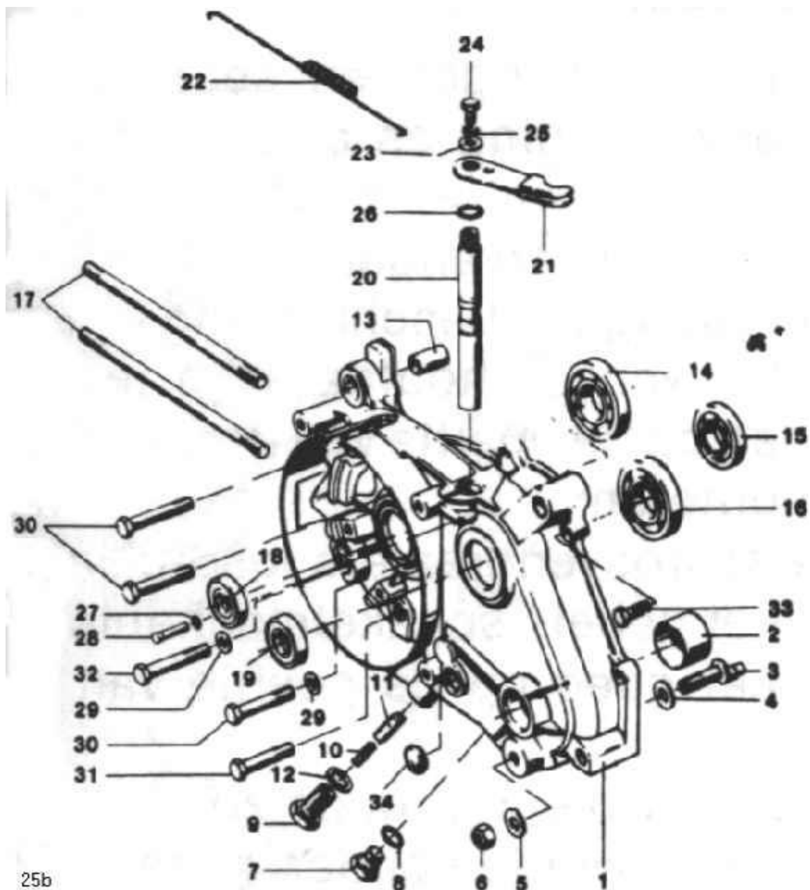
afb. 25b - carterhelft links (directe of hevelschakeling)
