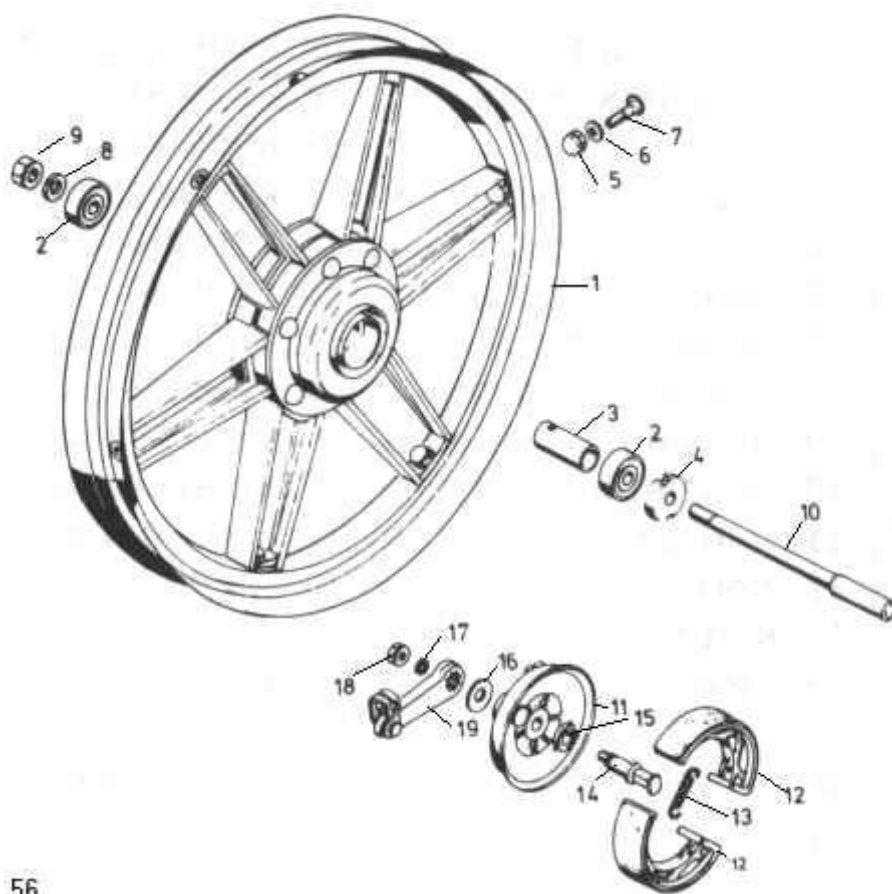
afb. 56 - voorsterwiel
