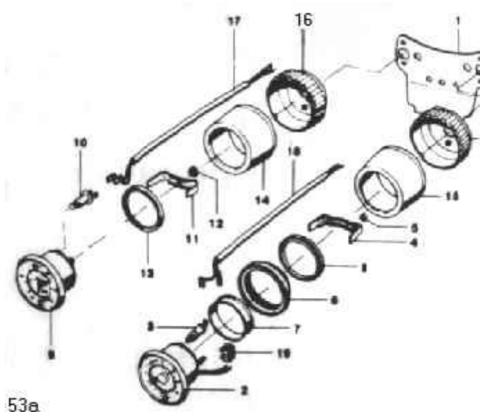
afb. 53a - opbouwteilers
