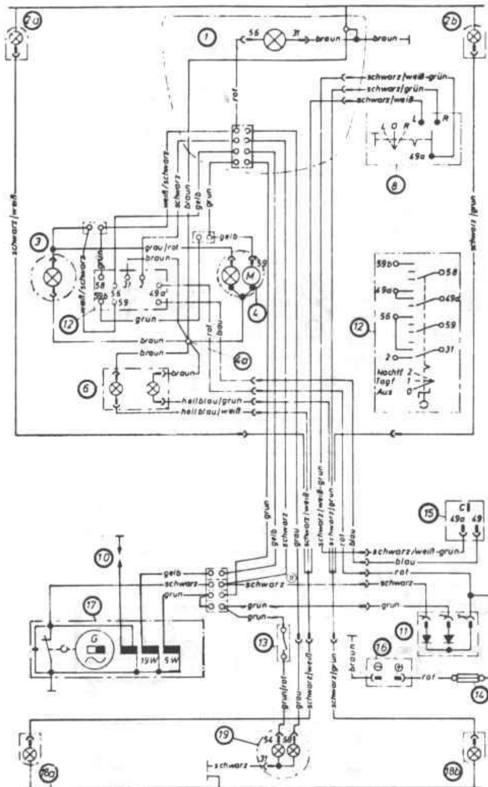
schema 6
