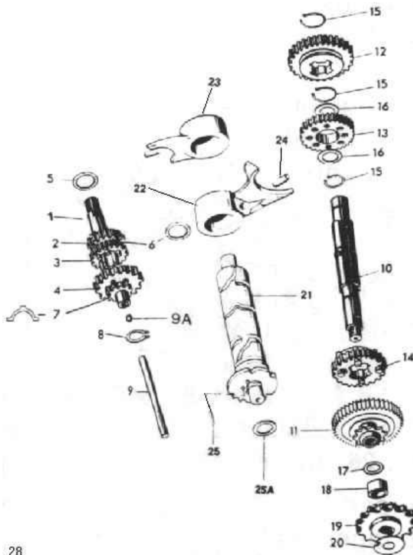
afb. 28 - 4 versnellingsbak (directe of hevelschakeling)
