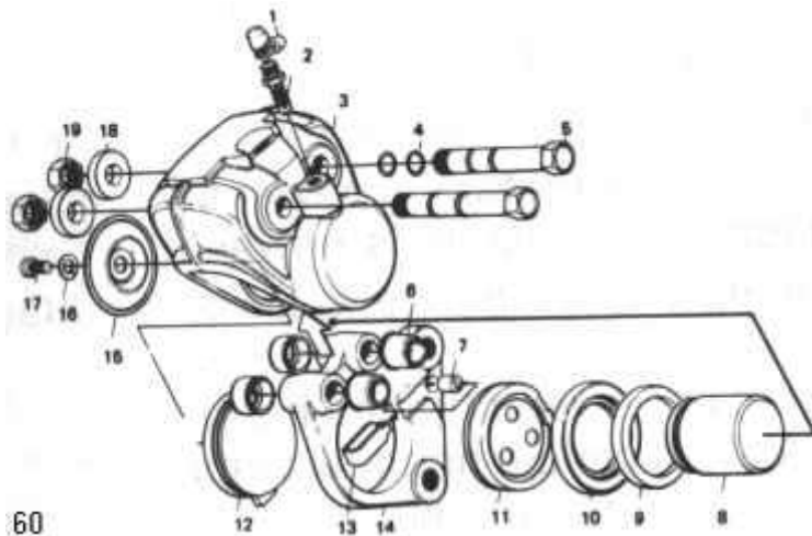
afb. 60 - schijfremklauw
