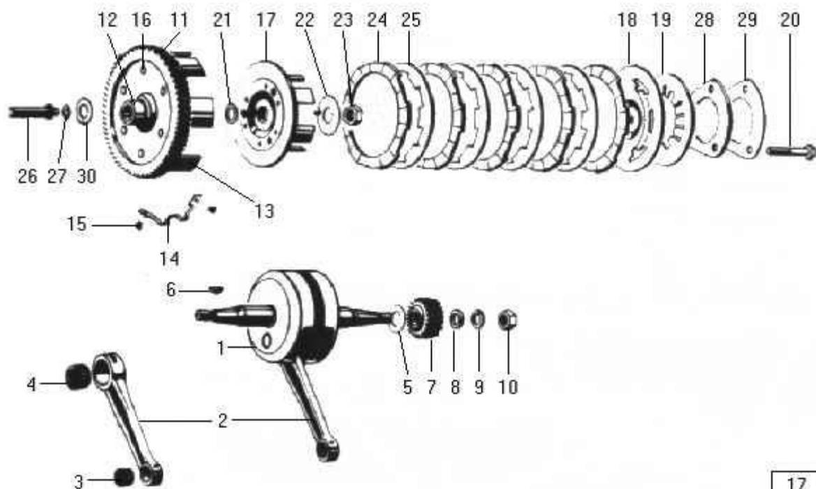
afb. 17 - krukas + koppeling
