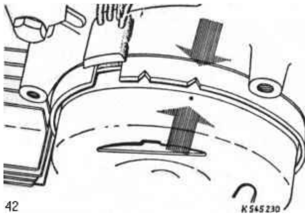
afb. 42 - Vliegwielmerktekens
