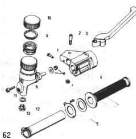
afb. 62 - rem/gashandle - schijfrem
