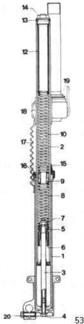
afb.53 - voorvork
