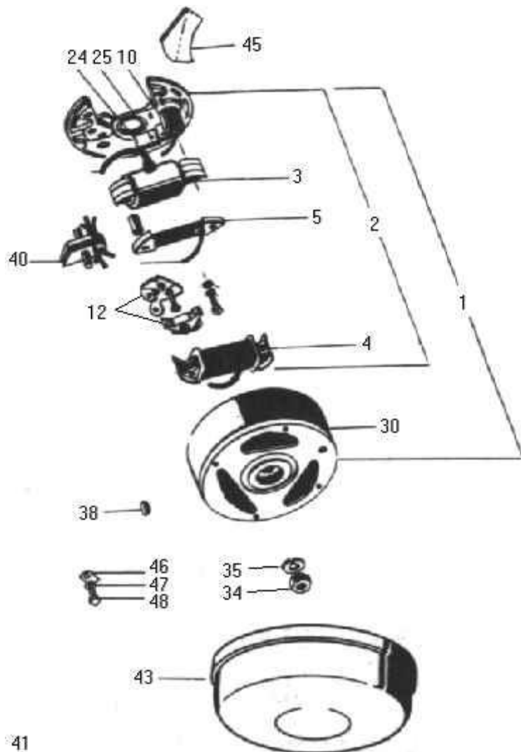
afb. 41 - Ontsteking 24 Watt
