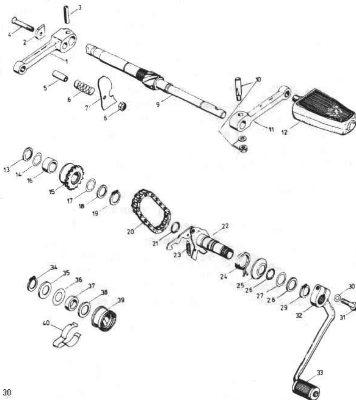
afb. 30 - Trapmechanisme (4 versn. directe schakeling)
