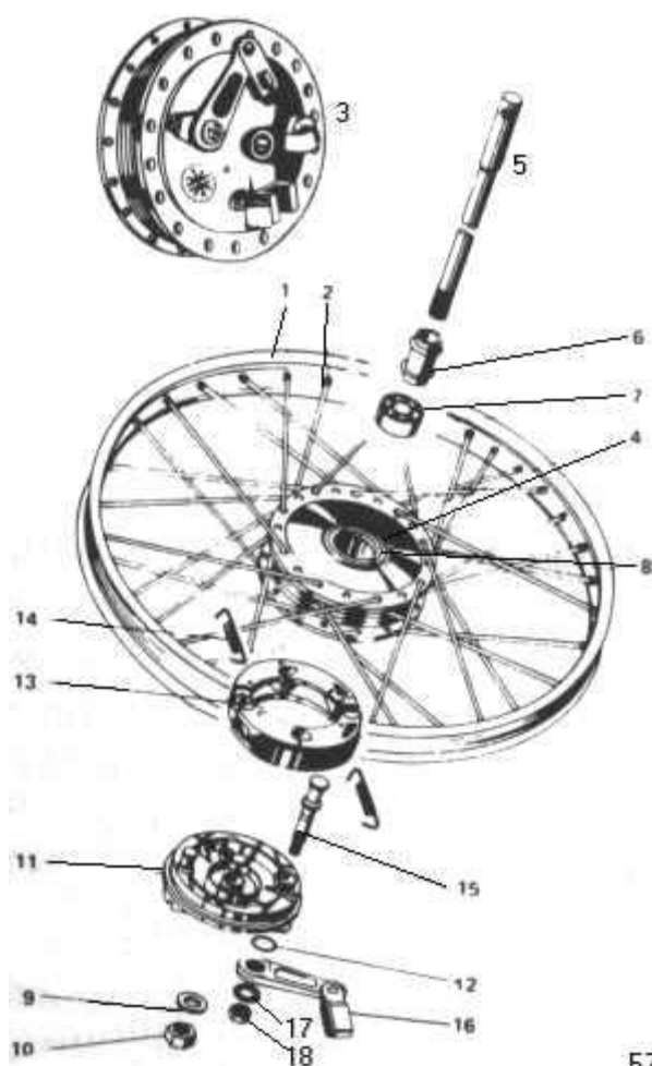
afb. 57 - voorspaakwiel
