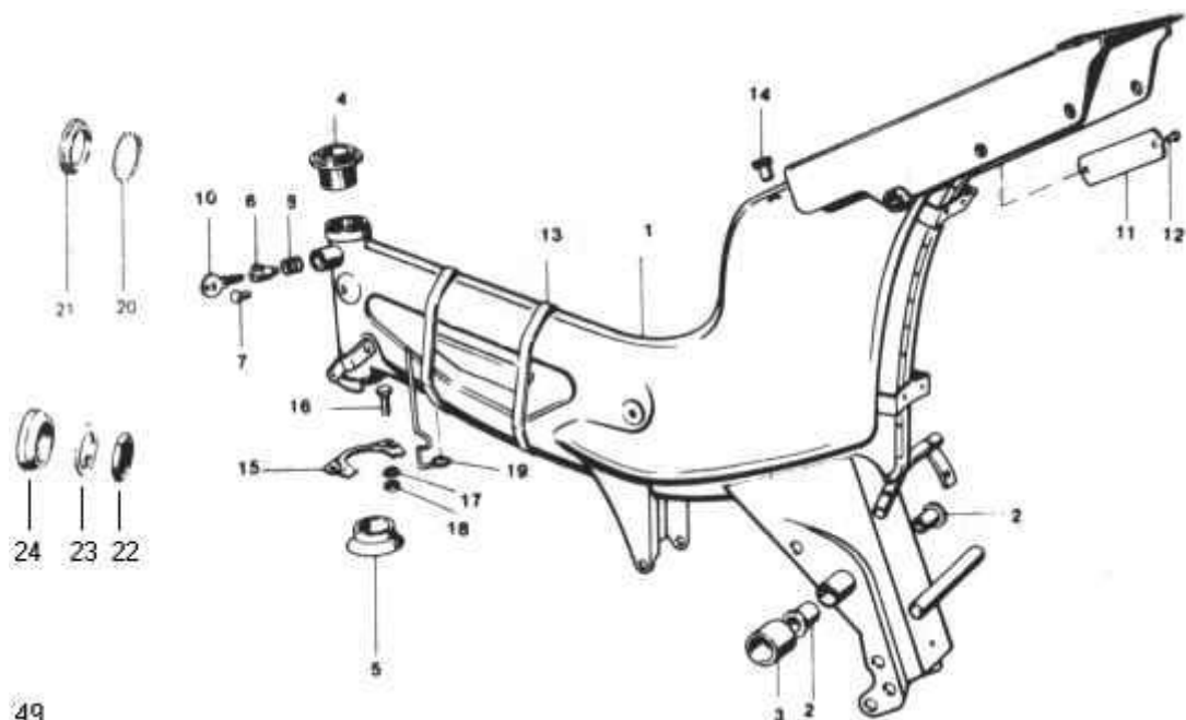
afb. 49 - frame
