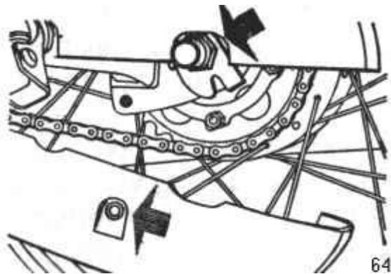
afb. 64 - afstellen vrije slag ketting
