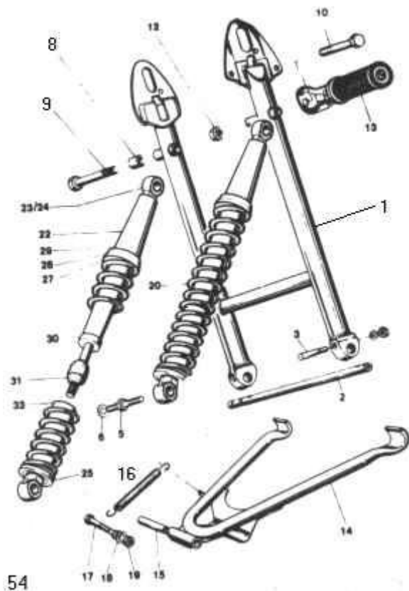
afb. 54 - achternork
