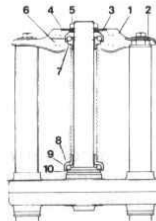
52 afb. 52 1. bovenste vorkplaat 2. stop (in binnenbuis) 3. stelring 4. vulring(en) 5. borgmoer 6. lagerkogel - 19x 7. lagercone boven 8. lagercup onder 9. lagerkogel - 19x 10. lagercone onder
